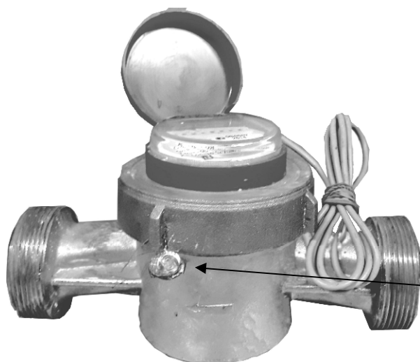
Рисунок 9 - Схема пломбировки от несанкционированного доступа, обозначение места нанесения знака поверки
